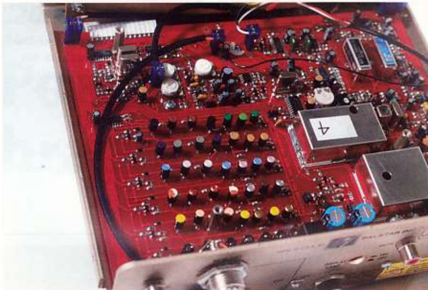
De bandfilters van de HF-350
